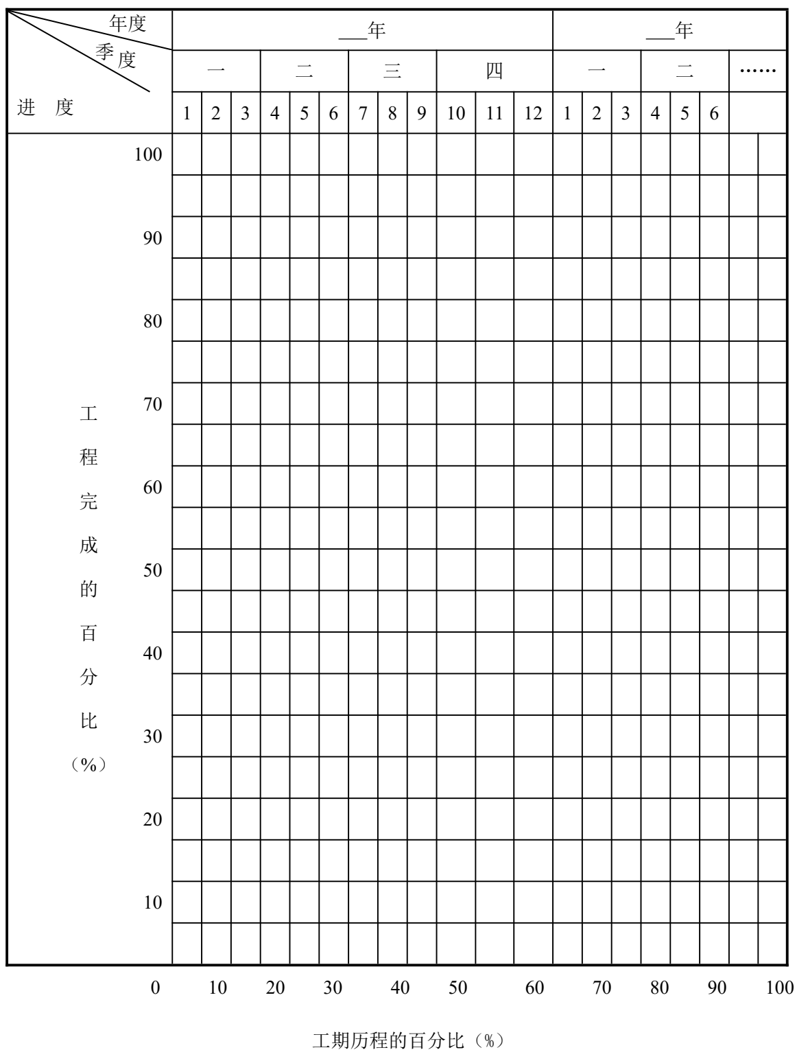
附表三 工程管理曲线
